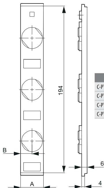
C-PTV-B D...195
