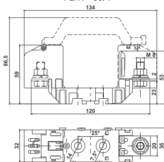
PLNV - 00/1
