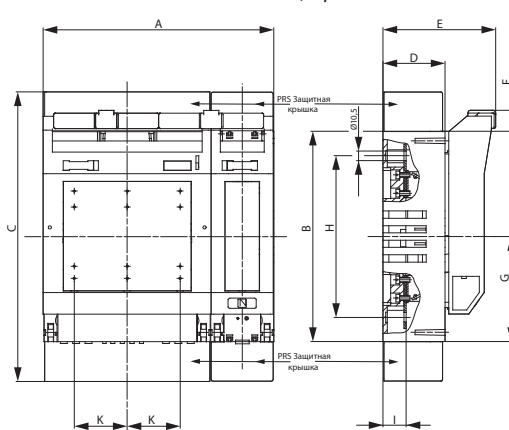
HVL 3
