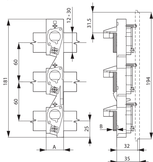
PTV-BD
