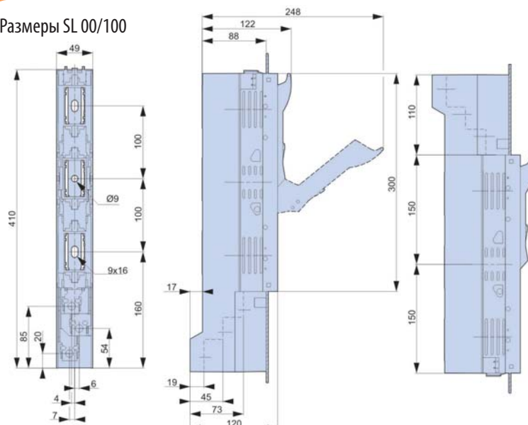
Размеры SL 00/185
