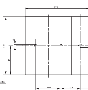
HVL 1
