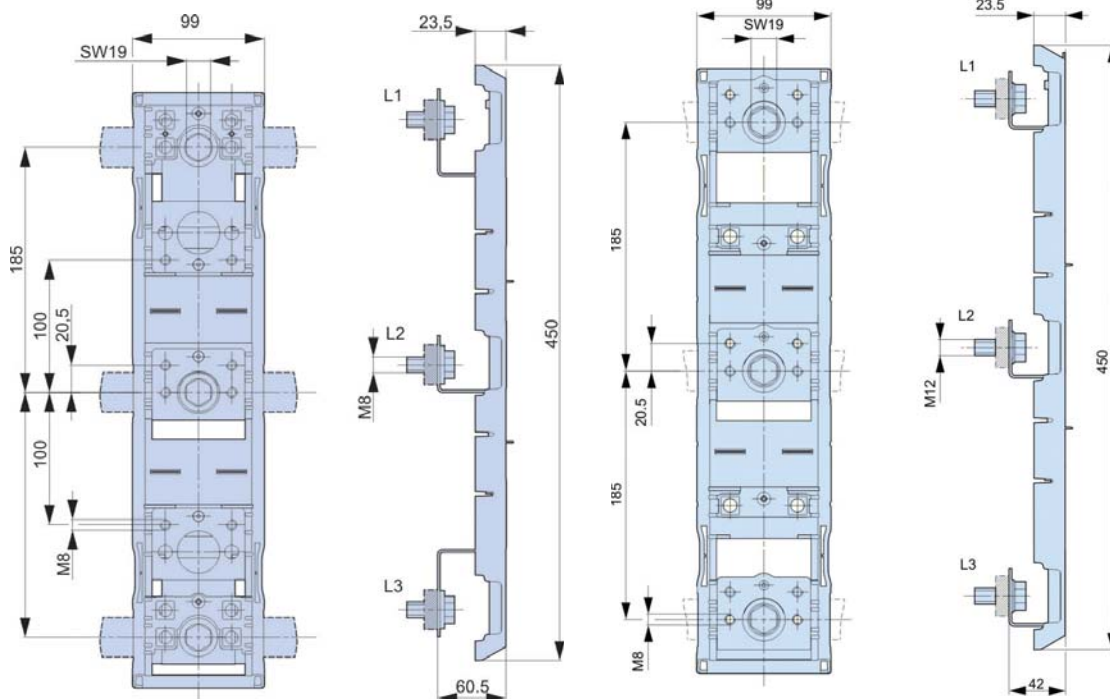
Адаптер 185-100/60
