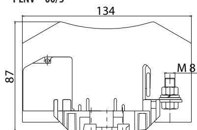
PLNV - 00/3
