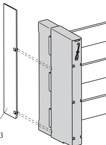
L-BBS-60/4
