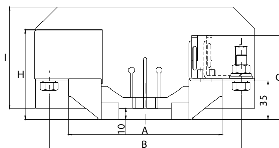
2PLNV - 1,2,3/3
