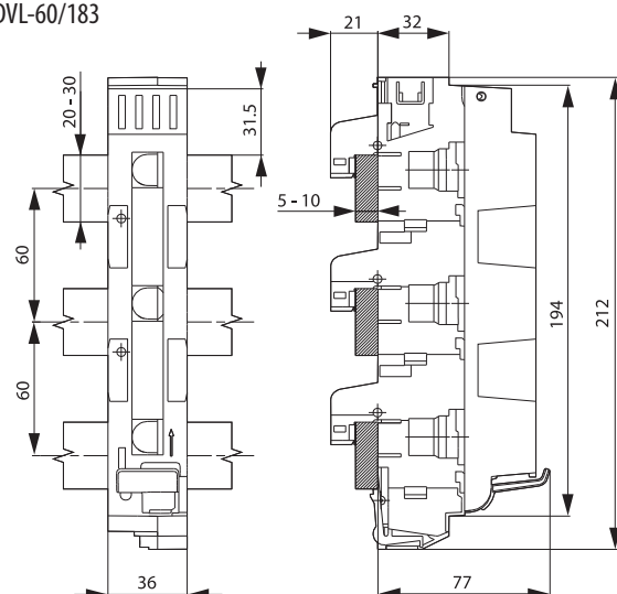
DVL-60/183
