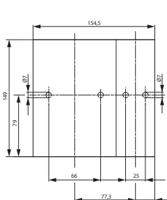
HVL 00
