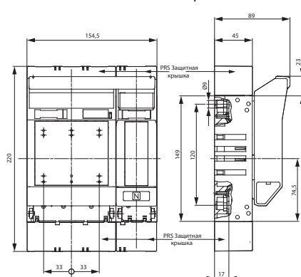
HVL 00 4p
