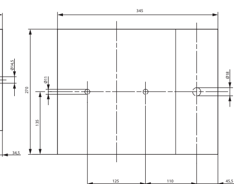
HVL 3
