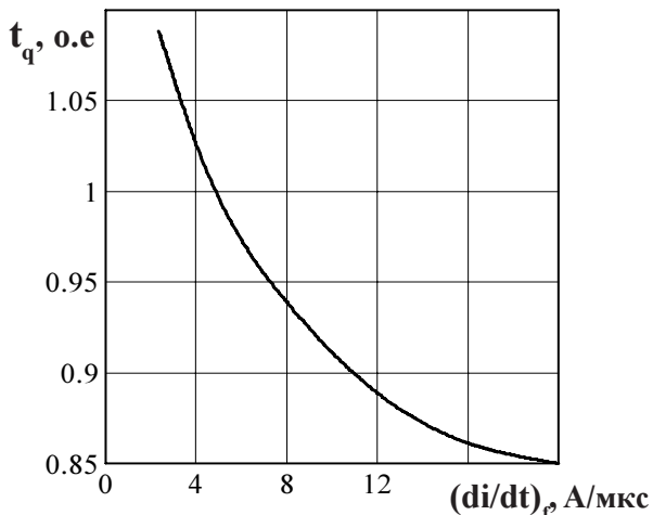
Рисунок 15 - Зависимость времени выключения t_q (о.е.) от скорости спада тока в открытом состоянии (di/dt)_p при T_{jm} = 125 \text{ } ^\circ\text{C} ; I_T = I_{T(AV)} ; U_R = 100 \text{ В} ; dU_D/dt = 50 \text{ В/мкс} ; U_D = 0,67 U_{DRM}
