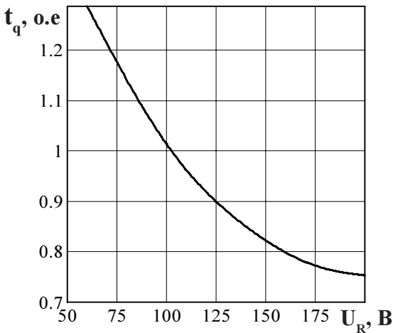
Рисунок 13 - Зависимость времени выключения t_q (о.е.) от обратного напряжения U_R при максимальной температуре перехода T_{jm} = 125 \text{ } ^\circ\text{C} ; I_T = I_{T(AV)} ; (di/dt)_f = 5 \text{ A/мкс} ; dU_D/dt = 50 \text{ В/мкс} ; U_D = 0,67 U_{DRM}
